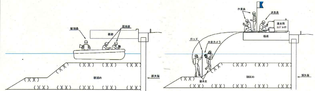
【作業船による調査 作業状況 断面図】
