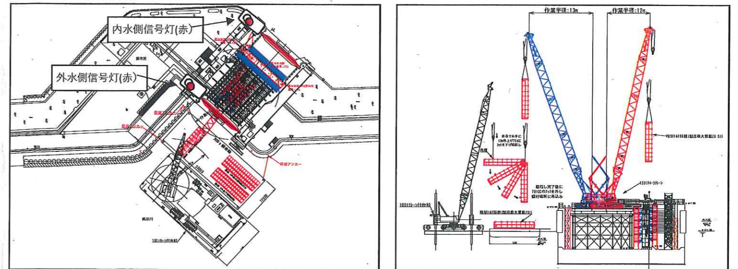
(2) クレーン配置計画
