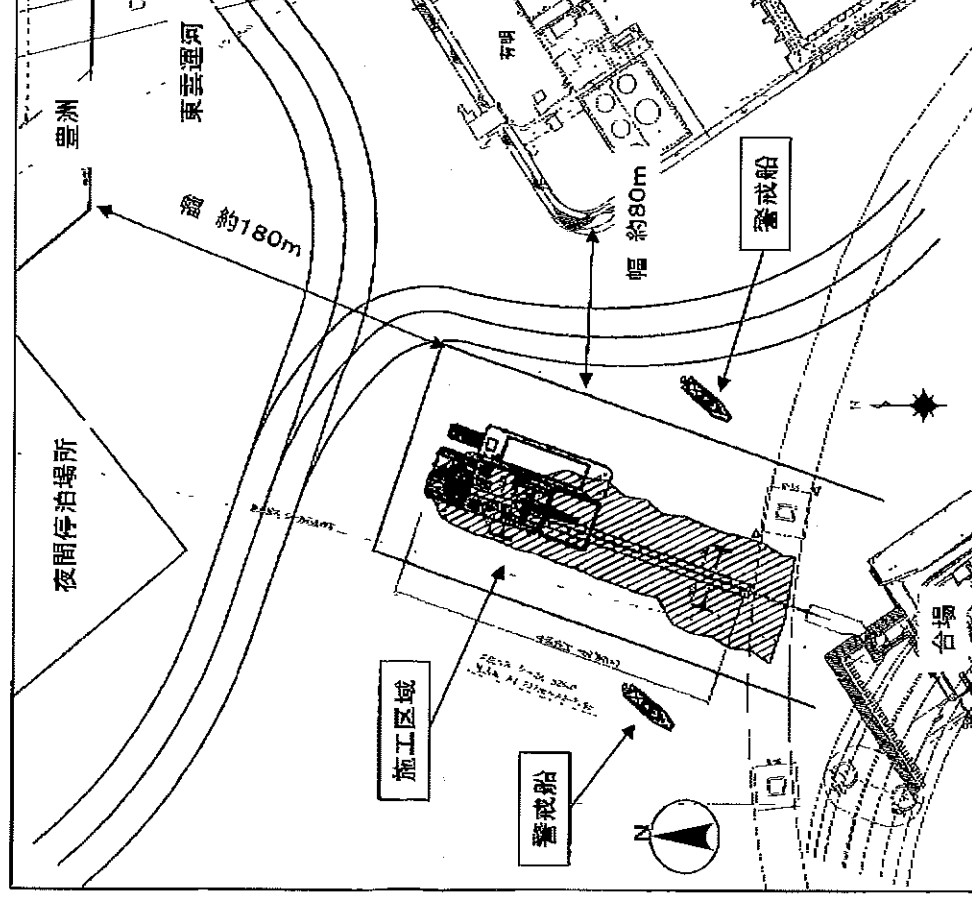
工事状況図
